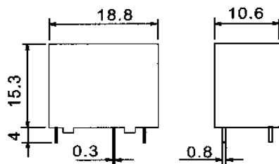
Dimensions 外型尺寸圖
