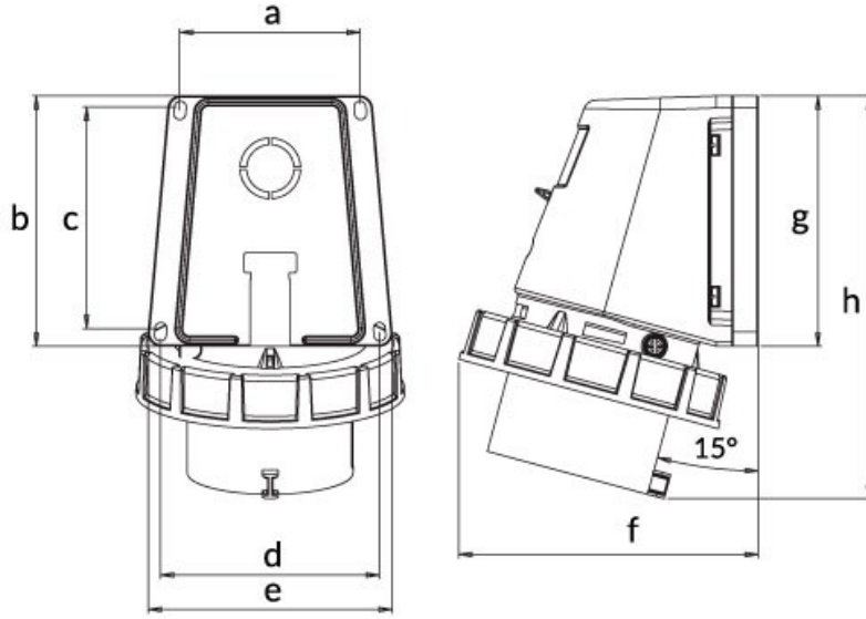
Ölçüler / Dimensions (mm)
